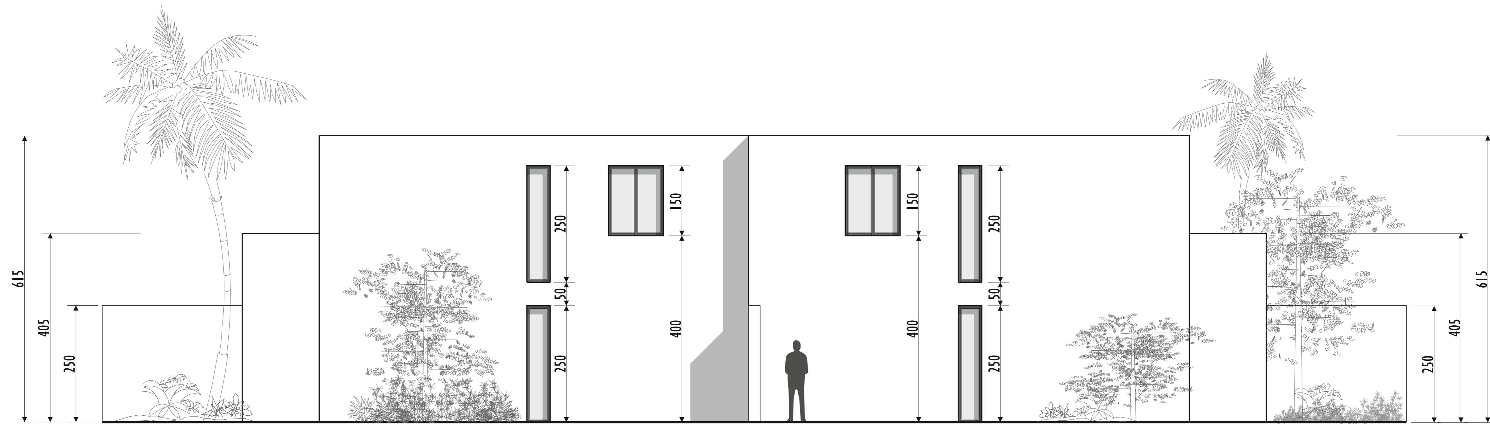
ELEVACION NORTE
