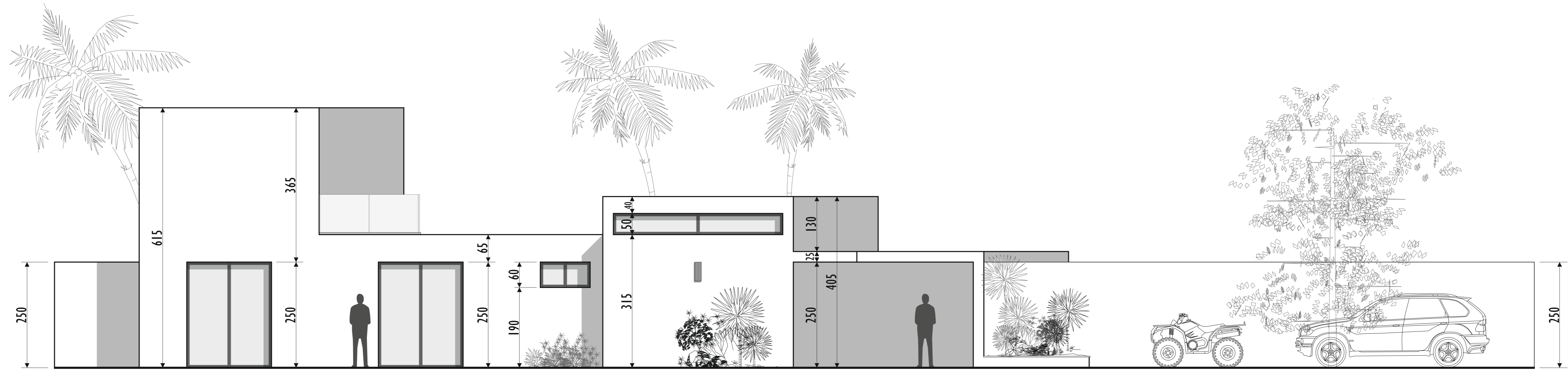
ELEVACION OESTE
